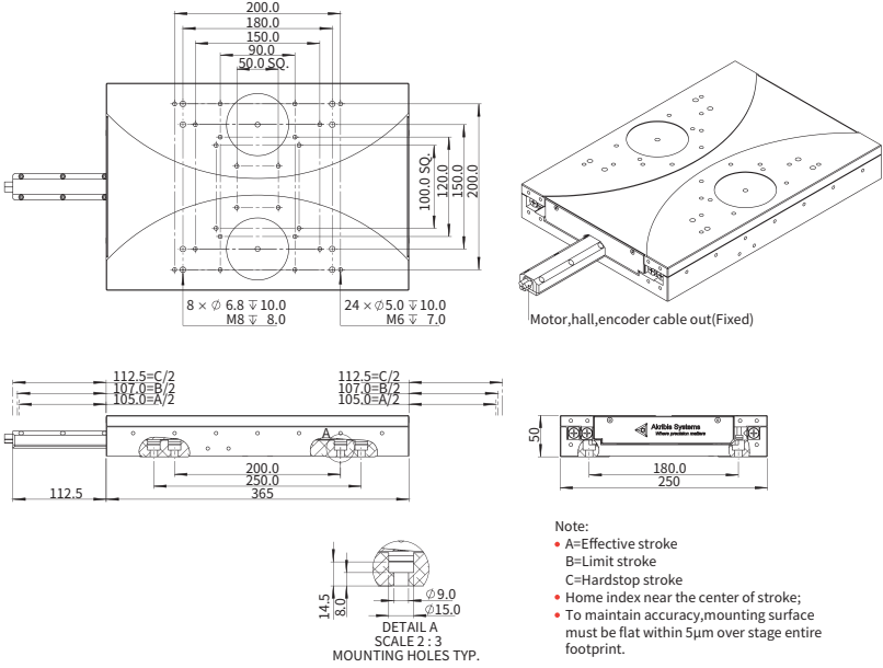
尺寸图
